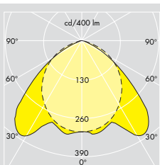
Titus Industri 2 x 49W T5 ULOR: 0% DLOR: 90% LOR: 90%
