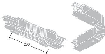
9. Fleksibelt vinkelstykke, XTS 23 (Flex coupler)
