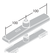
11. Pendelbeslag hvid, SP41 (Trackfixing middel)
