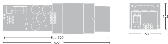
Separat el-udstyr er forsynet med spole, fasekondensatorer, klemrække og sikring. Alle komponenter er monteret på pladen.
