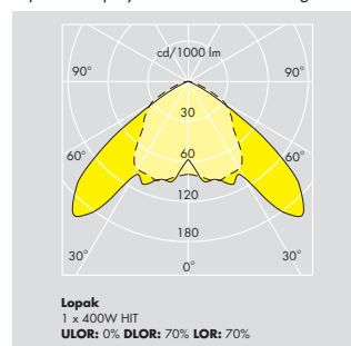
Lopak med polycarbonat afskærmning
