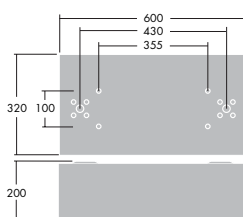
Lopak med wiregitter
