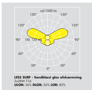
Less m/sandblæst glas afskærmning
