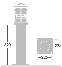
Aluminiumstolpe med fodflange
