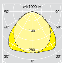
Indus RDx bredstrålende 2x49W T5 ULOR: 0% DLOR: 90% LOR: 90%
