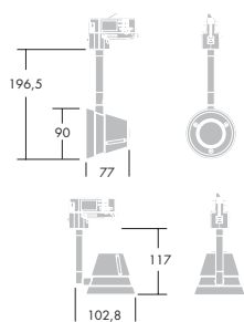
Graffiti S, PAR 16 og QR-CBC for 3-faset kontaktskinne
