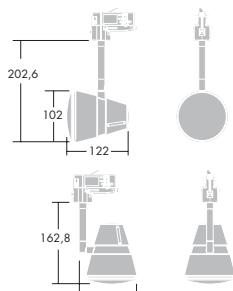
Graffiti S, PAR 20/30 for 3-faset kontaktskinne
