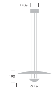
Uden uplight 600 (1 x 150W QT)
