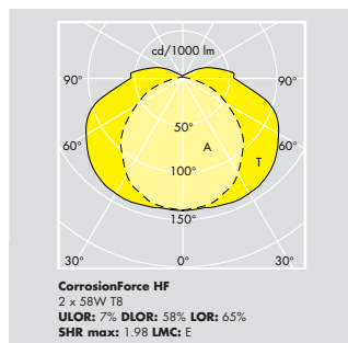
T-rørs version
