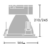
Udskæring Ø190, Chalice 190V TC-D 13/18W (Internt el-udstyr)
