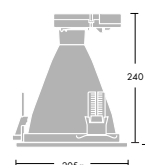
Udskæring Ø190, Chalice 190V 18W, TC-D/TC-D EL 26W, TC-D EL 32W, 42W
